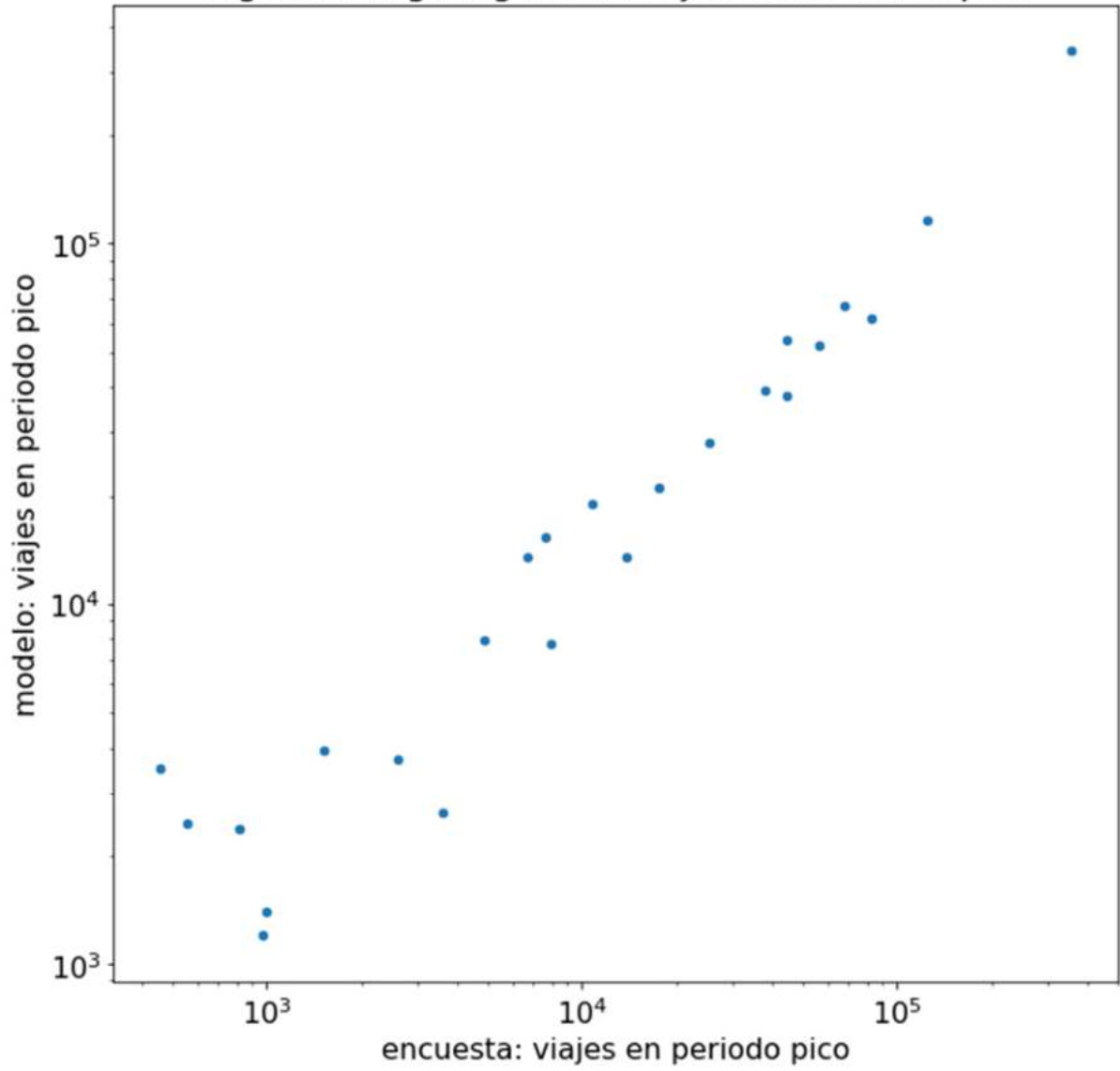
Illustration 15. Calibración de los flujos entre municipios: buble chart regresión log / log de los flujos entre municipios
