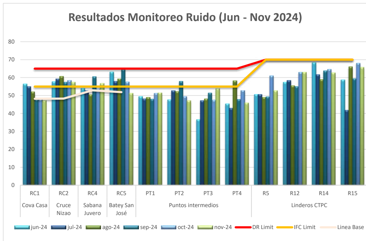
Gráfico. 1 Comportamiento de los niveles de ruido en los últimos 6 meses
