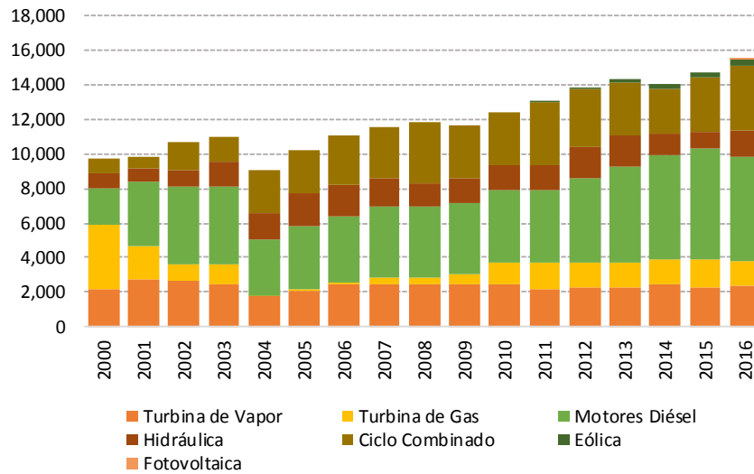
Gráfico 10 Producción de Electricidad por Tipo de Tecnología, 2000 - 2016 (Cifras expresadas en GWh)
