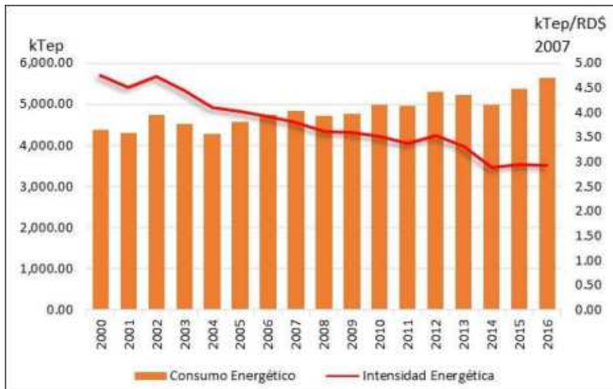
Gráfico 5 Intensidad Energética Total vs Consumo Energético 7
