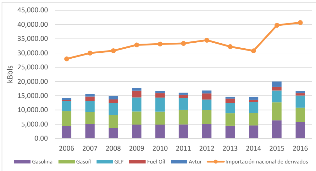
Gráfico 17 Productos derivados de petróleo importados por REFIDOMSA vs. Importación nacional de derivados, 2016. (Unidades expresadas en miles de barriles, kbbl)
