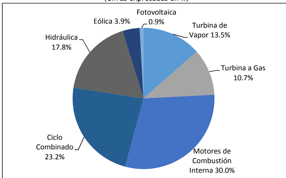
Gráfico 7 Capacidad Instalada del SENI por tipo de Tecnología, 2016 (Cifras expresadas en %)
