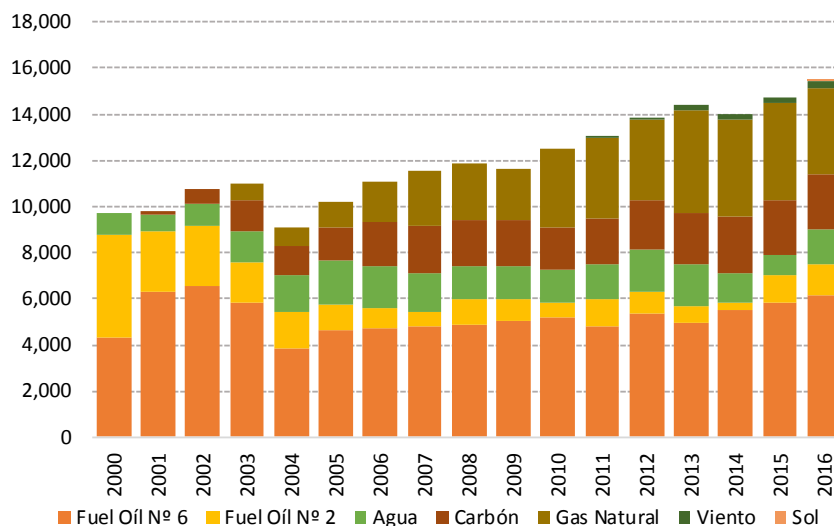
Gráfico 9 Producción de Electricidad por fuente, 2000 - 2016 (Cifras expresadas en GWh)
