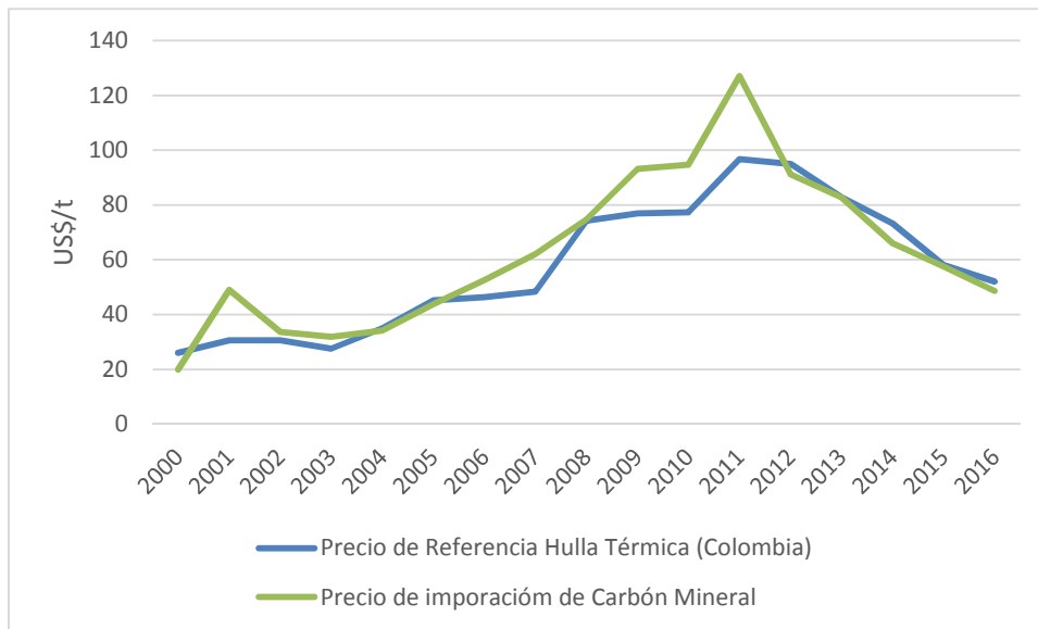
Gráfico 20 Precio de referencia de exportación de Hulla Térmica de Colombia vs. Precios de adquisición del Carbón Mineral, 2000-2016. (Unidades expresadas en dólares americanos por tonelada, US$/t)
