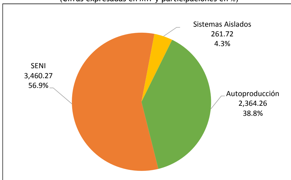
Gráfico 6 Capacidad Instalada Nacional, 2016 (Cifras expresadas en MW y participaciones en %)
