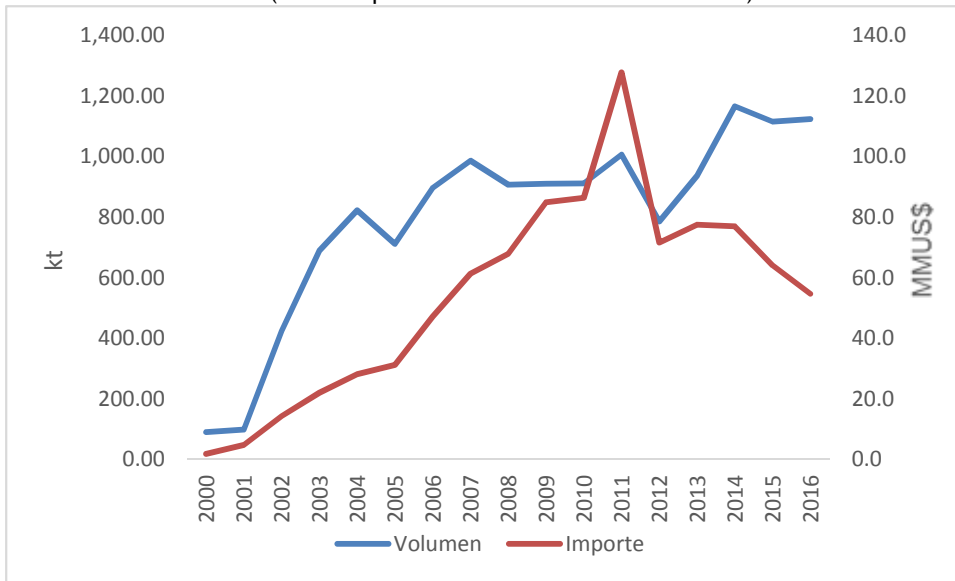
Gráfico 19 Importaciones nacionales de carbón mineral, 2000 - 2016. (Cifras expresadas en las unidades indicadas)
