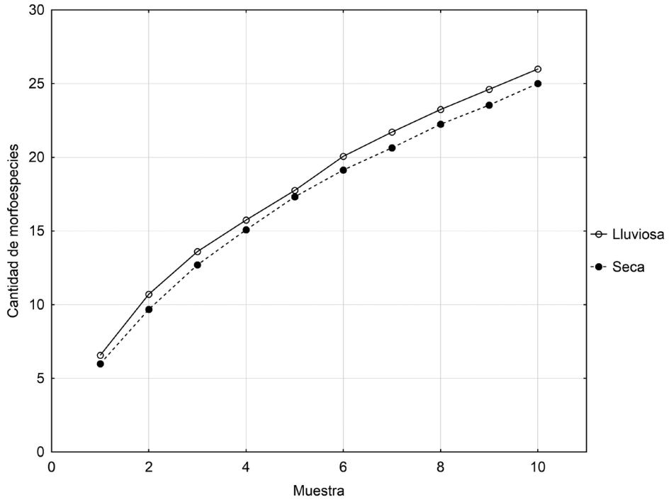
Figura 1. Curvas de acumulación de especies ajustadas a la ecuación de Clench. Temporada lluviosa: Sobs= 26, R 2 = 0.994, a= 6.68, b= 0.16, pendiente= 0.99. Temporada seca: Sobs= 25, R 2 = 0.997, a= 6.13, b= 0.15, pendiente= 0.98.
