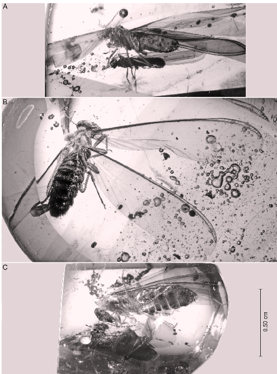
Fig. 21. Photomicrographs of imagoes of Nasutitermes spp. in Dominican amber; all are holotypes. A. N. ampliocolatus , n. sp., AMNH DR10-1680. B. N. incisus , n. sp., AMNH DR-PB263. C. N. mediocolatus , n. sp., AMNH DR14-643.
