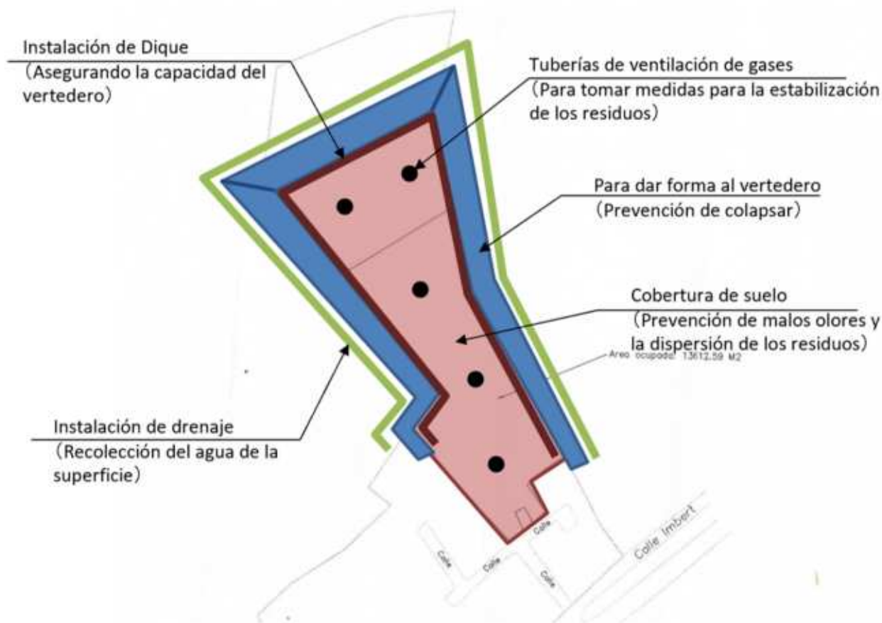
Figura 26: Esquema conceptual del cierre para la preparación del proyecto
