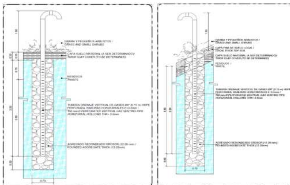
Figura 14: Instalación de tubería venteo de gases en terreno plano (izquierda) e inclinado (derecha)
