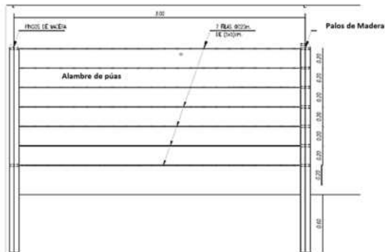
Fuente: Diseño de un plan de Manejo Integral para los residuos sólidos en la MAGSD, Nippon Koei-Kokusai Kogyo, BID, 2013 Figura 21: Ejemplo de una verja típica con alambres de púas
