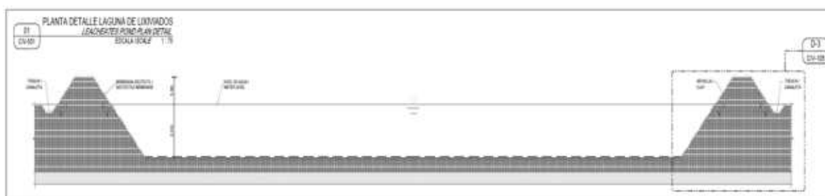
Figura 16: Sección transversal de una laguna de lixiviados
