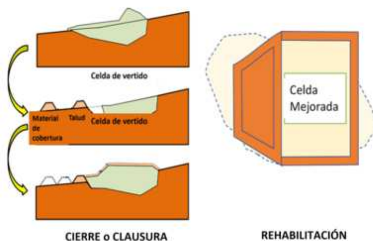
Figura 5: Diagrama sobre el concepto de Cierre y Rehabilitación de un SDF Existente.
