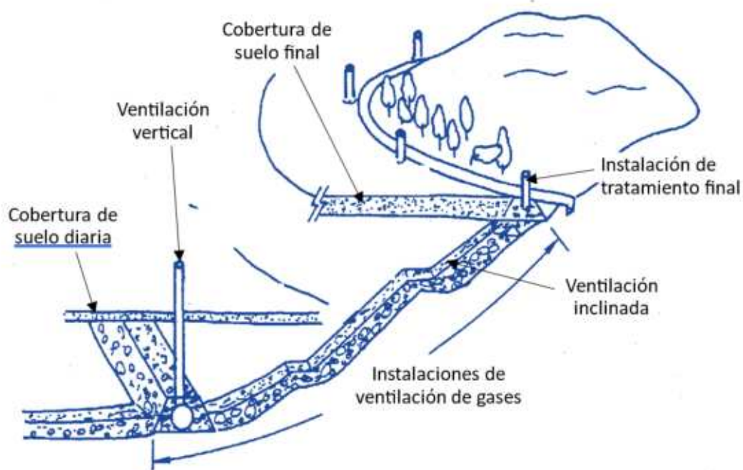
Figura 36: Dibujo Conceptual instalaciones para ventilación de gases
