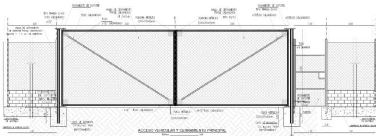
Figura 17: Portón de acceso vehicular típico de un SDF
