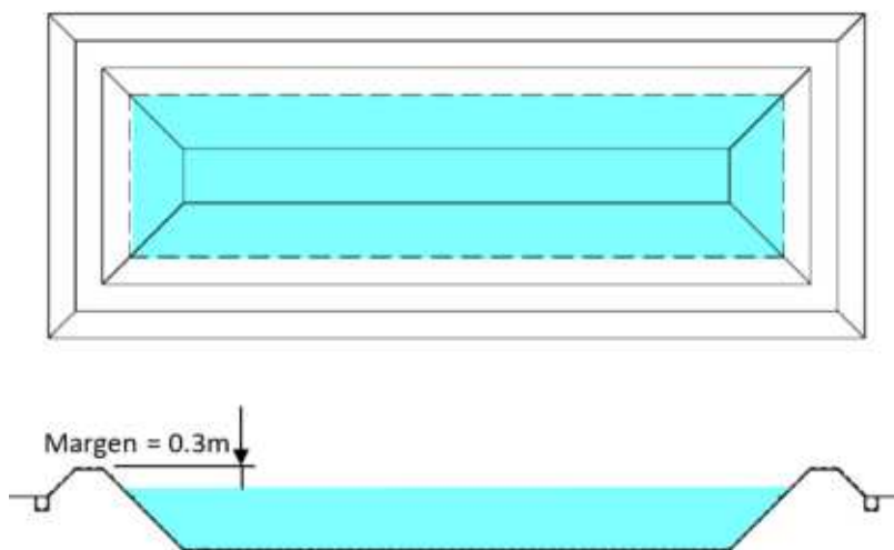
Figura 34: Imagen de una laguna de lixiviados
