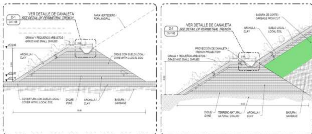
Figura 22: Instalación de banqueta en área de residuos (izquierda) y banqueta en la base (derecha)
