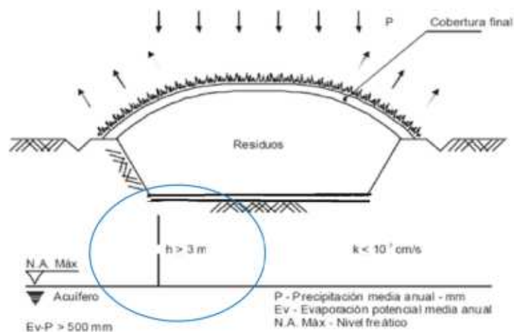
Figura 12: Esquema condiciones climatológicas e hidrológicas favorables.
