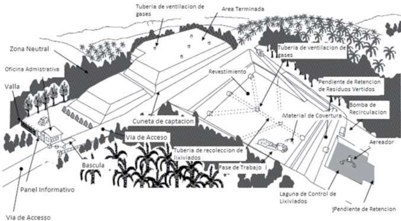
Figura 14: Relleno sanitario con Nivel 4 de construcción
