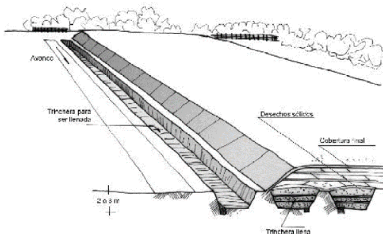
Figura 7: Conformación de una celda por el método combinado.
