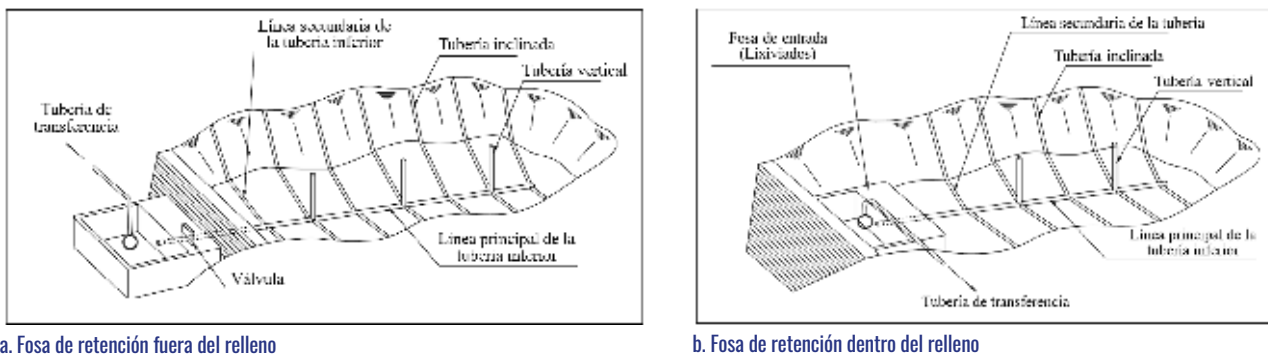
Figura 28: Concepto de instalación de recolección de lixiviados
