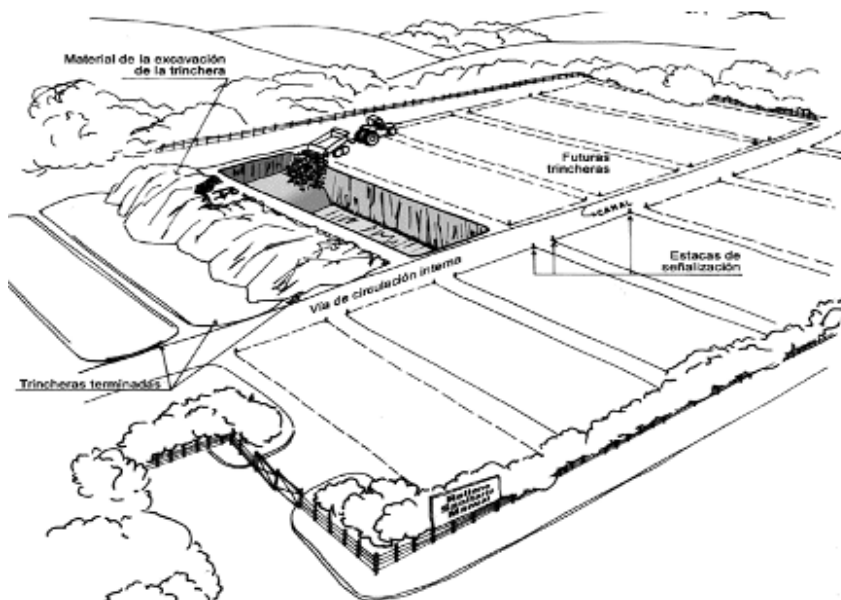
Figura 5: Vertido por el Método de Trinchera
