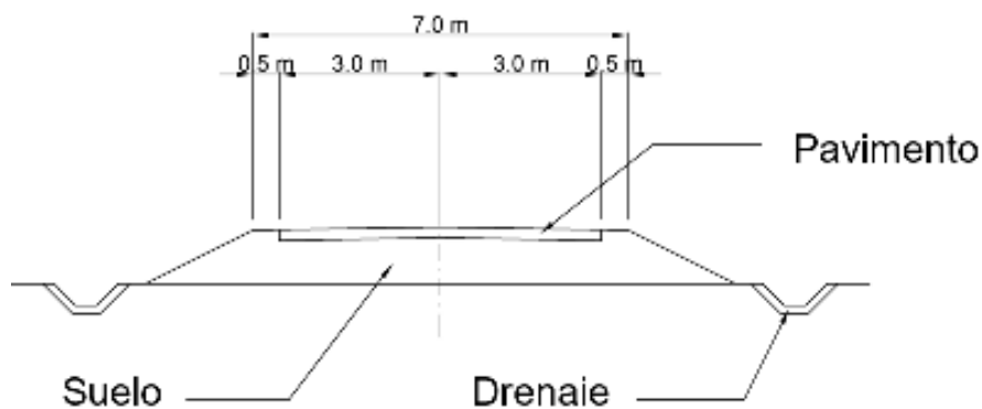
Figura 40: Esquema de una sección transversal un camino de acceso
