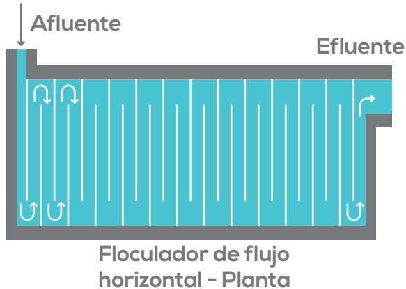
Floculador (Tebaco, 2018)
