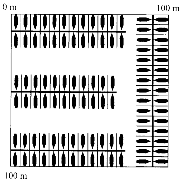
Figura 5.5. Representación esquemática del número de embarcaciones que pueden distribuirse en un Marina de 10,000 m 2 .
