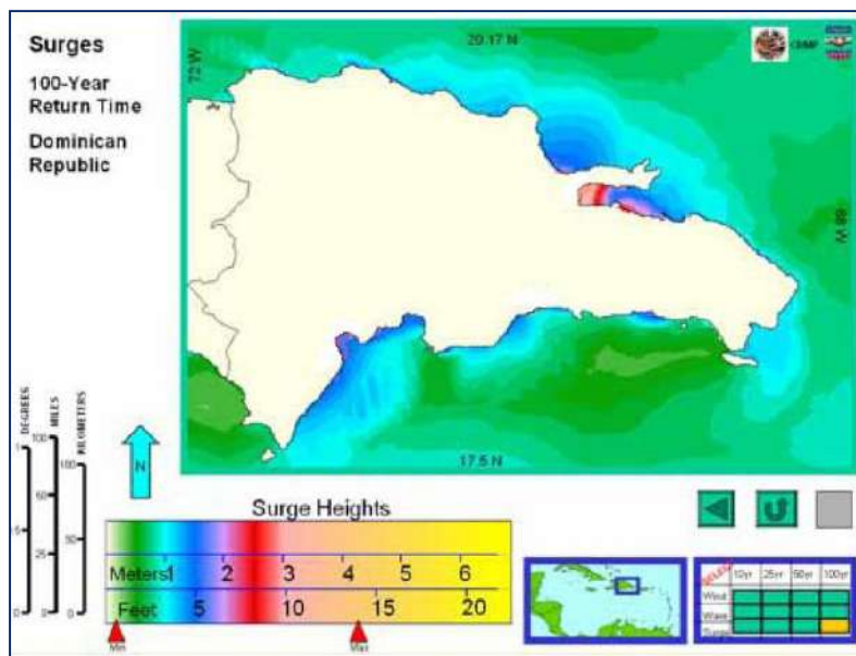
Figura 10. Altura significativa de las olas durante la ocurrencia de eventos meteorológicos extremos con probabilidades de no excedencia de 100 años. Fuente: CRP/USAID (2005).
