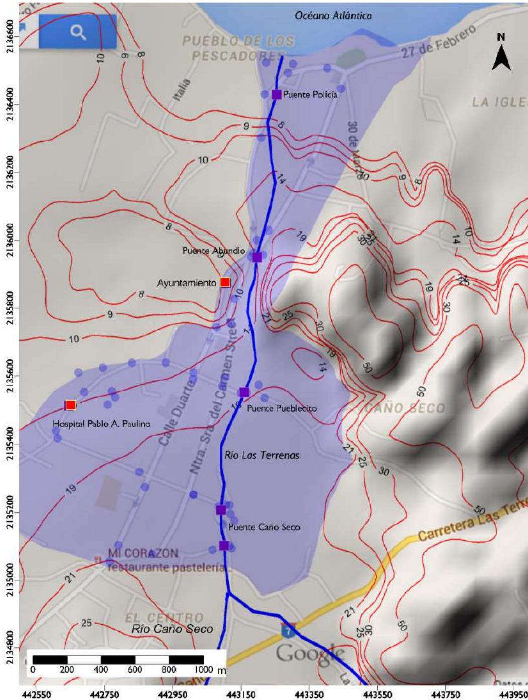
Figura 8. Mapa preliminar de inundación de la zona urbana de Las Terrenas (zona azul) delimitada partir de puntos georreferenciados (círculos azules) sobre las curvas de alturas (línea roja) del modelo topográfico digital. Se indican los puentes (cuadros morados) y algunos sitios de interés (cuadros rojos). Fuente: ICMA/AMLT.
